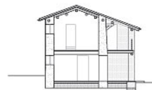
sezione c-c'
